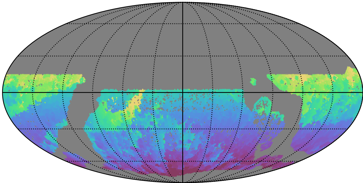
baseline_v3.2_10yrs WFD r band: Min HA
