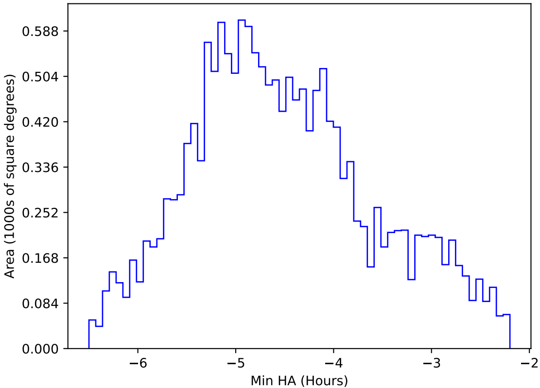
baseline_v3.2_10yrs WFD r band: Min HA
