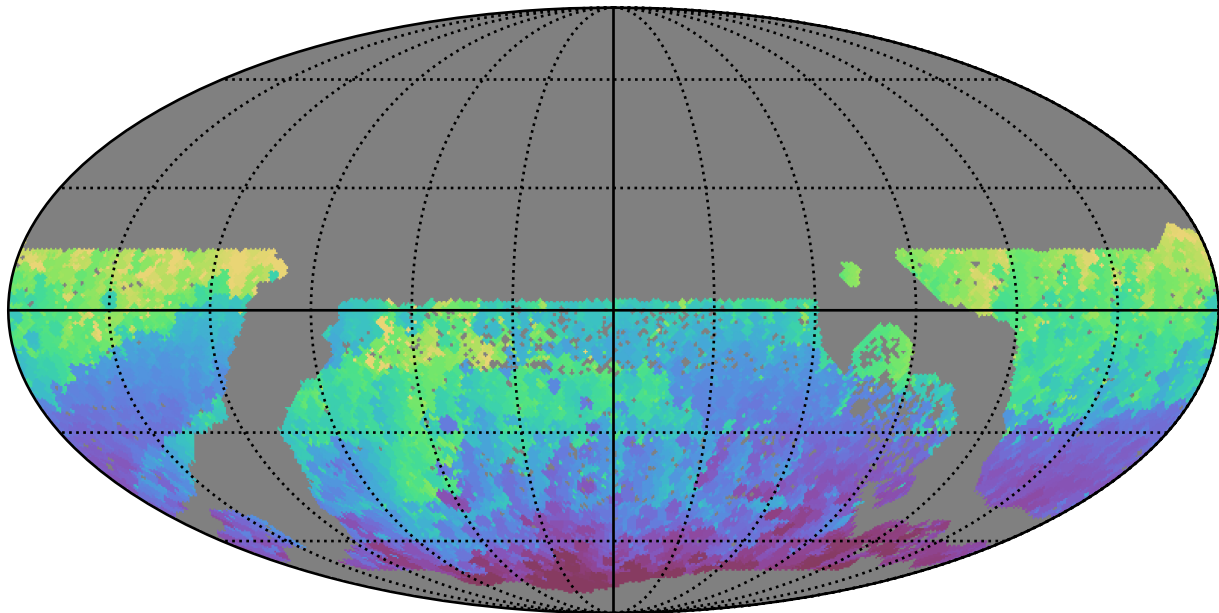
baseline_v3.2_10yrs WFD i band: Min HA
