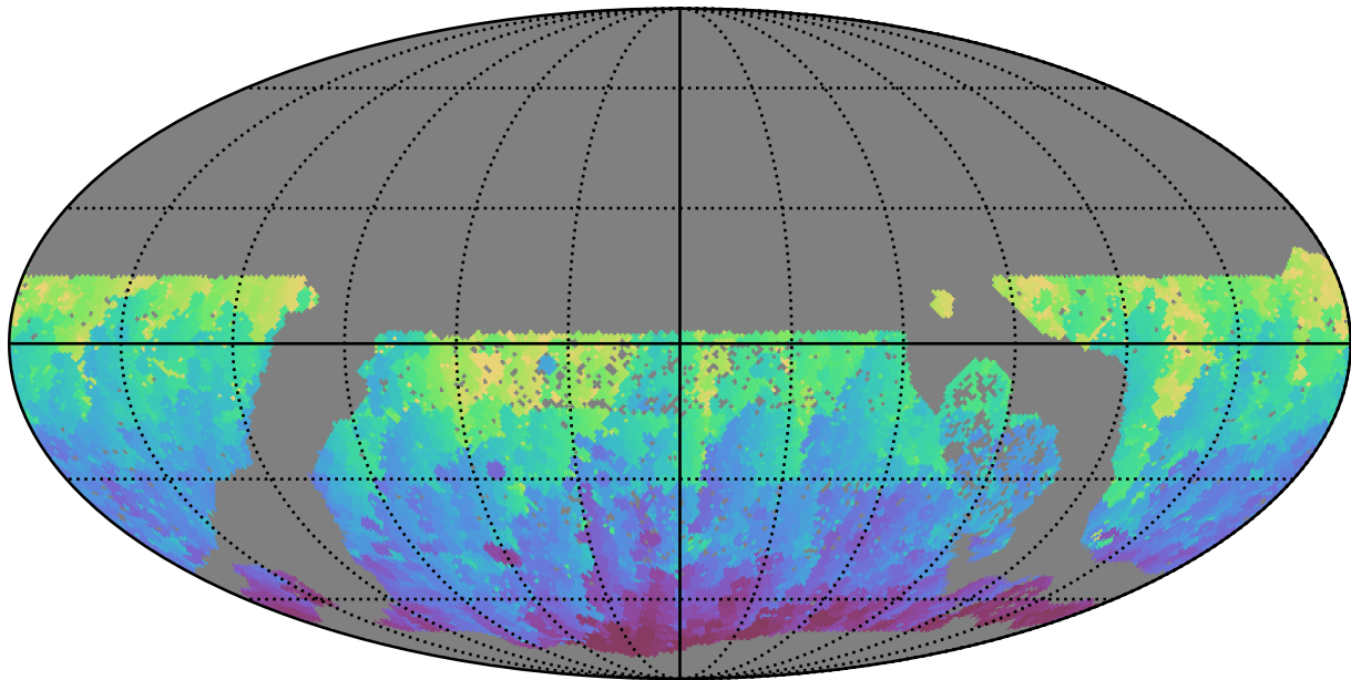
baseline_v3.2_10yrs WFD g band: Min HA
