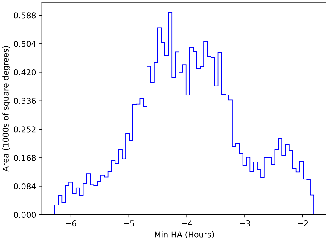
baseline_v3.2_10yrs WFD g band: Min HA
