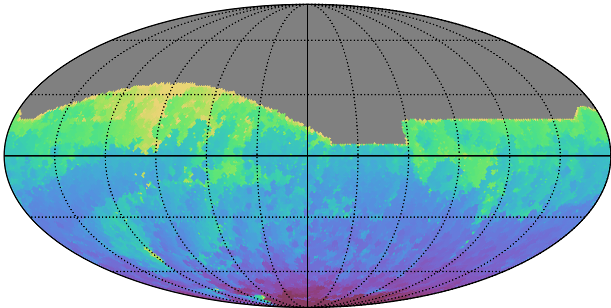
baseline_v3.2_10yrs All sky z band: Min HA
