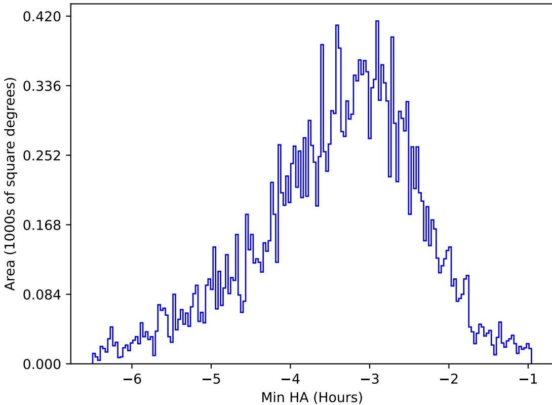
baseline_v3.2_10yrs All sky y band: Min HA
