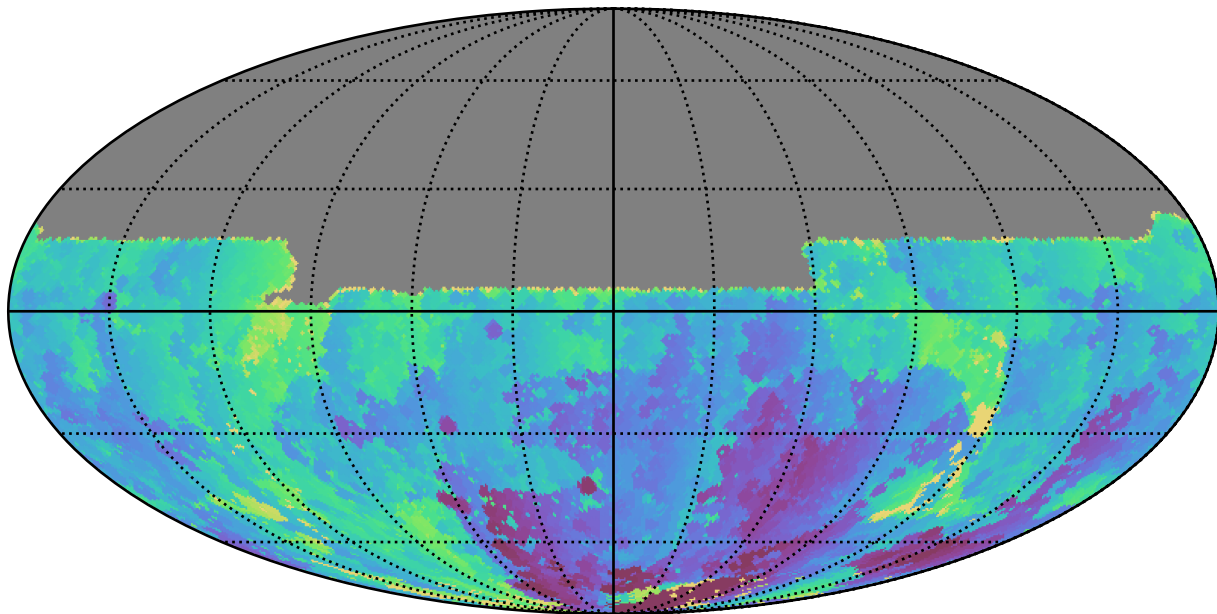
baseline_v3.2_10yrs All sky u band: Min HA
