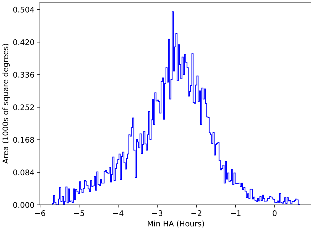
baseline_v3.2_10yrs All sky u band: Min HA
