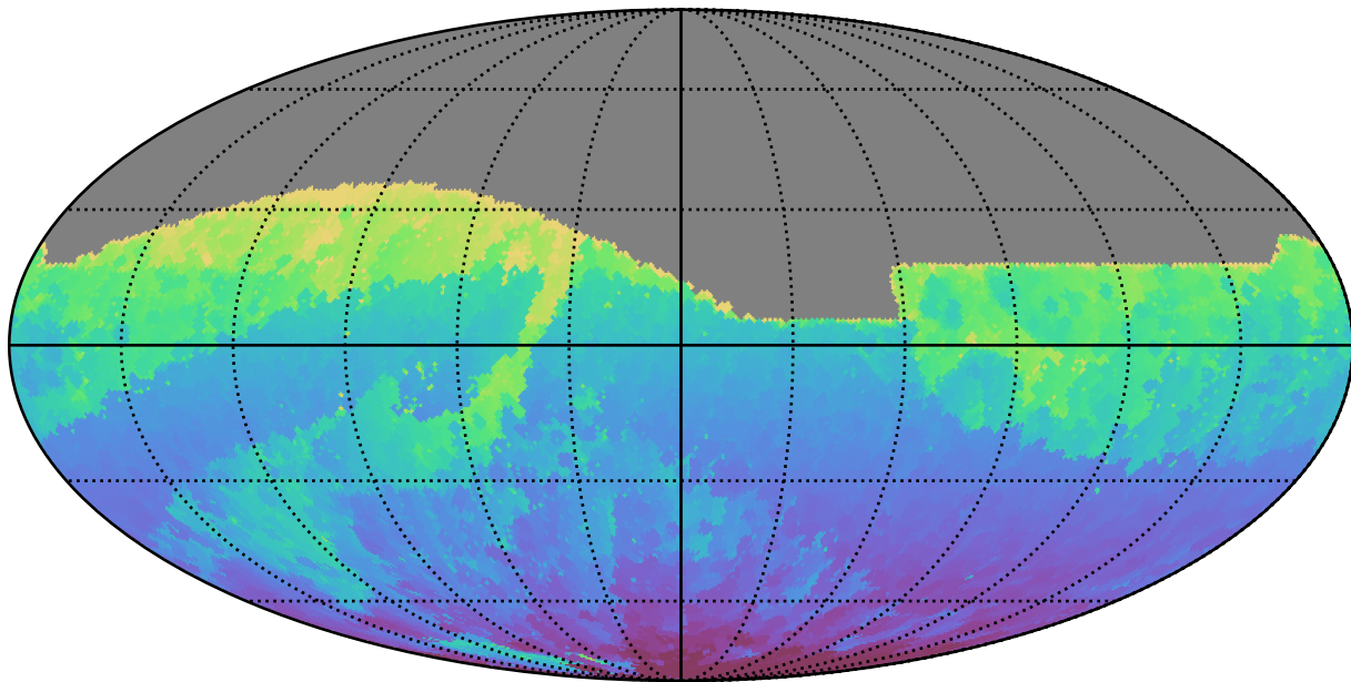
baseline_v3.2_10yrs All sky r band: Min HA
