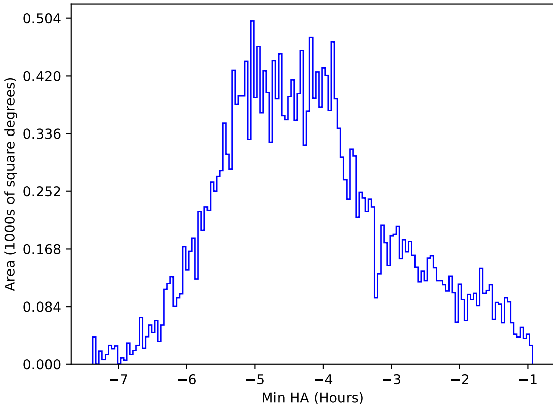
baseline_v3.2_10yrs All sky r band: Min HA
