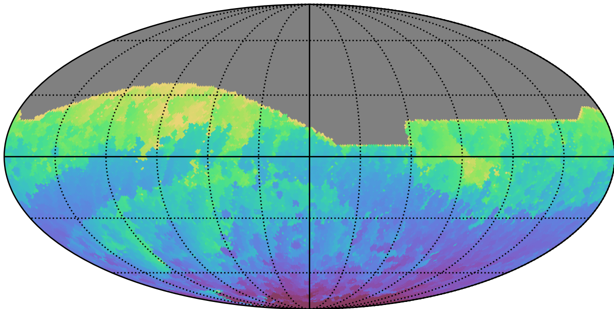
baseline_v3.2_10yrs All sky i band: Min HA
