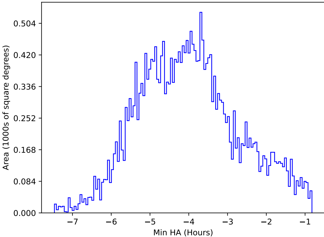
baseline_v3.2_10yrs All sky i band: Min HA
