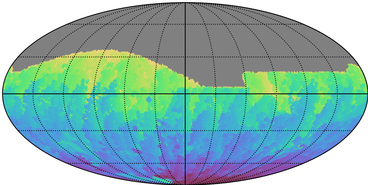
baseline_v3.2_10yrs All sky g band: Min HA
