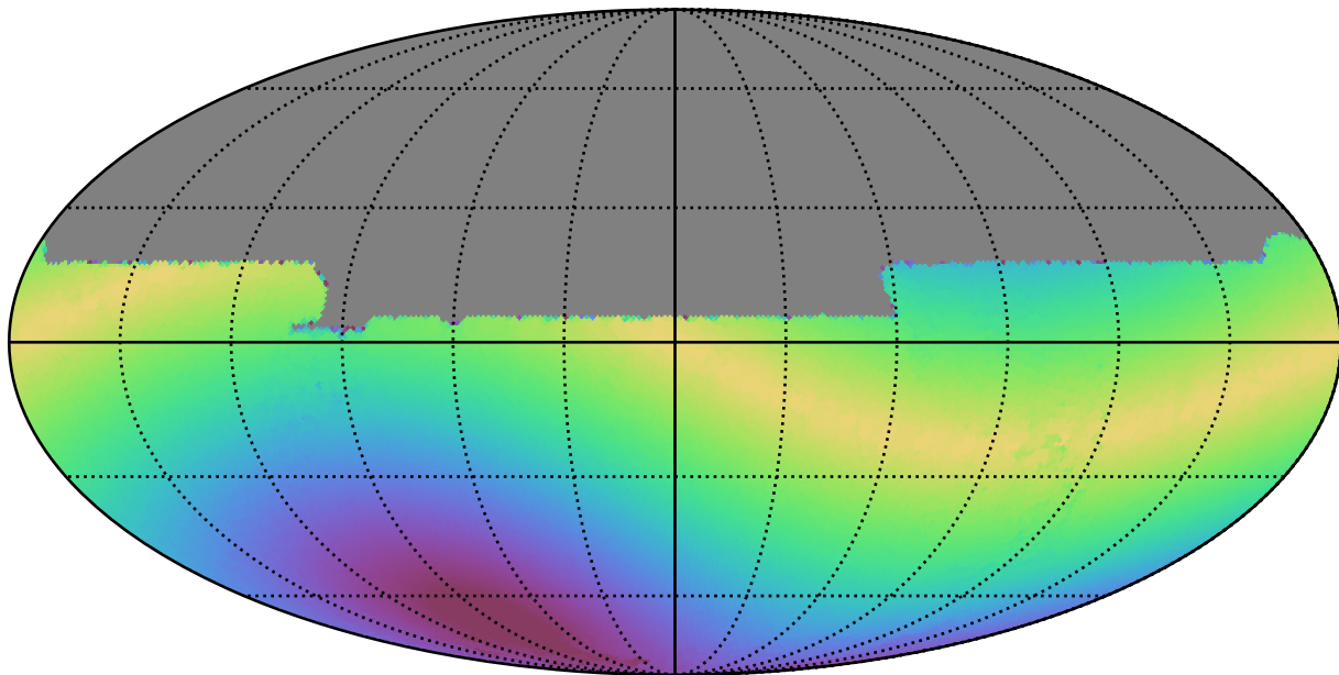
baseline_v3.2_10yrs All sky y band: Max solarElong
