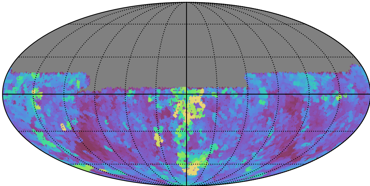
baseline_v3.2_10yrs Yr 1 y band: Max seeingGeom
