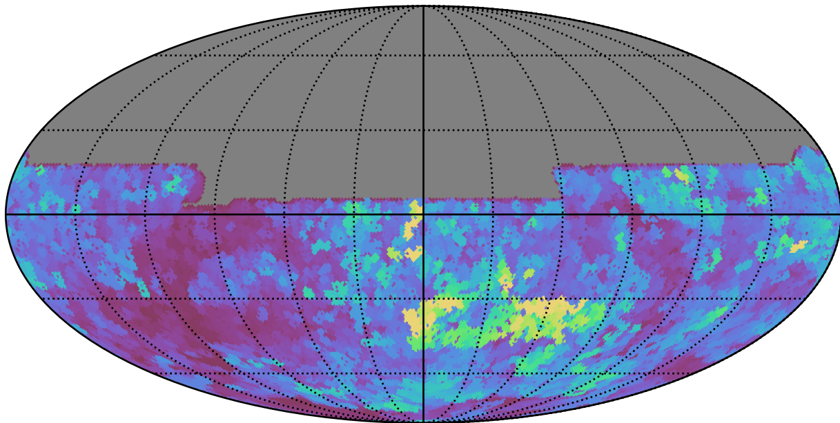
baseline_v3.2_10yrs All sky y band: Max seeingEff
