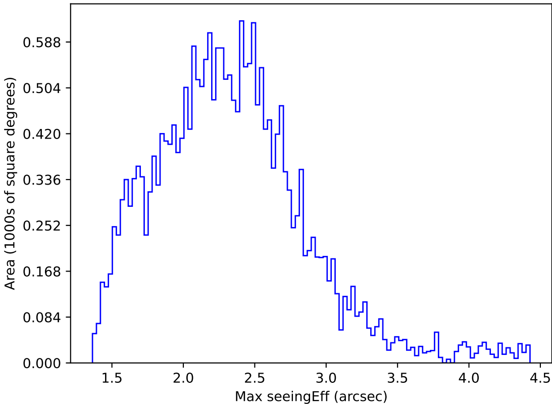
baseline_v3.2_10yrs All sky y band: Max seeingEff
