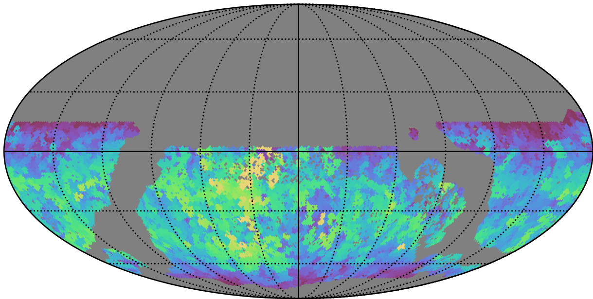
baseline_v3.2_10yrs WFD y band: Max saturation_mag
