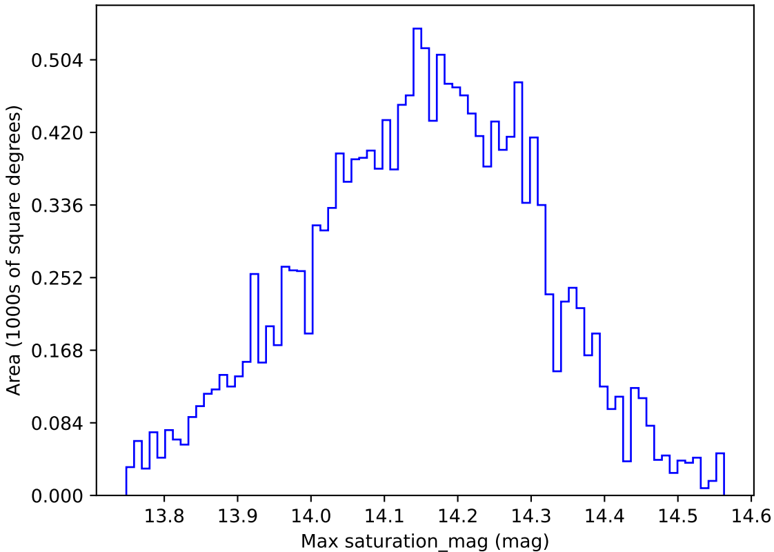
baseline_v3.2_10yrs WFD y band: Max saturation_mag
