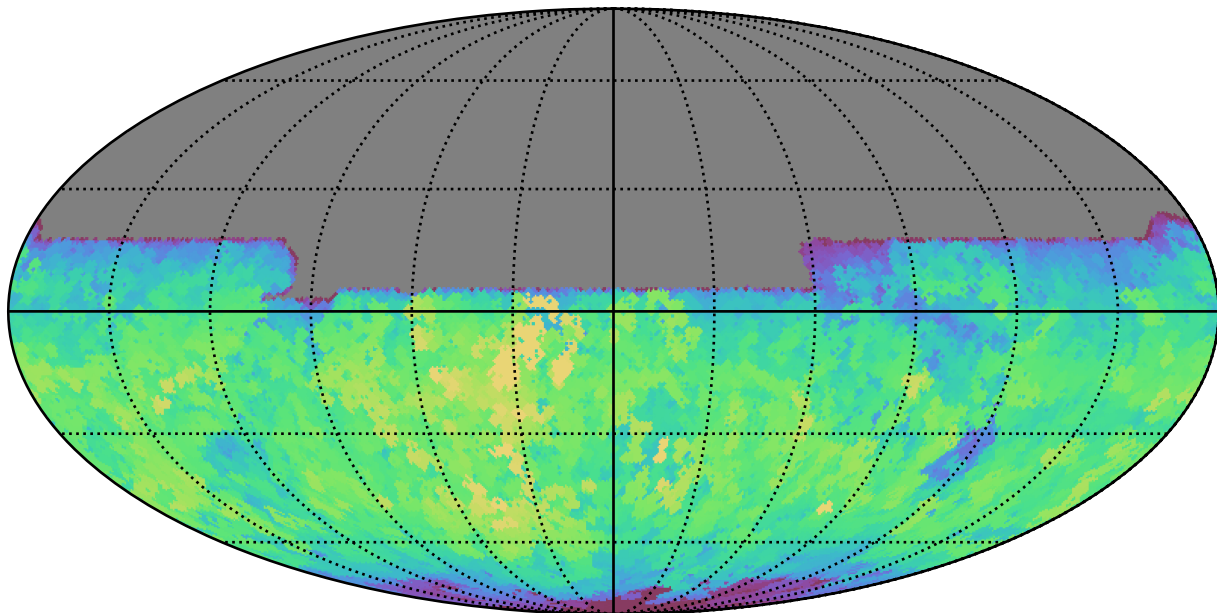
baseline_v3.2_10yrs All sky y band: Max saturation_mag
