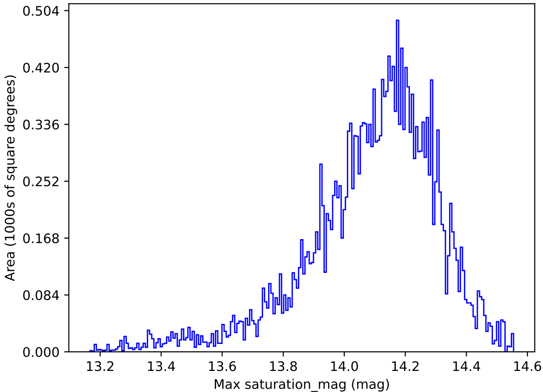
baseline_v3.2_10yrs All sky y band: Max saturation_mag
