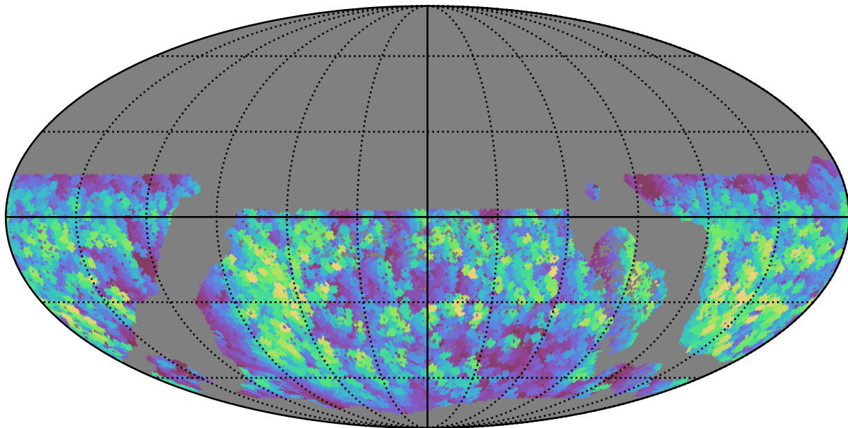
baseline_v3.2_10yrs WFD y band: Max normairmass
