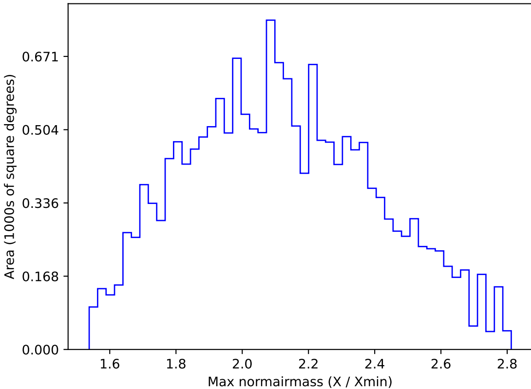
baseline_v3.2_10yrs WFD y band: Max normairmass
