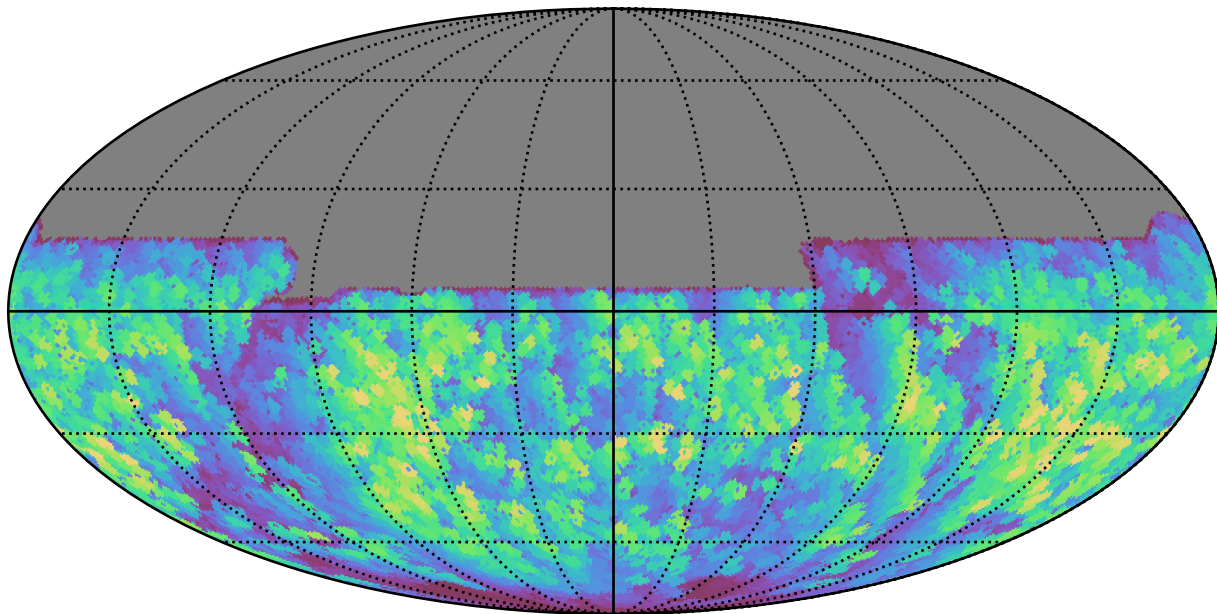
baseline_v3.2_10yrs All sky y band: Max normairmass
