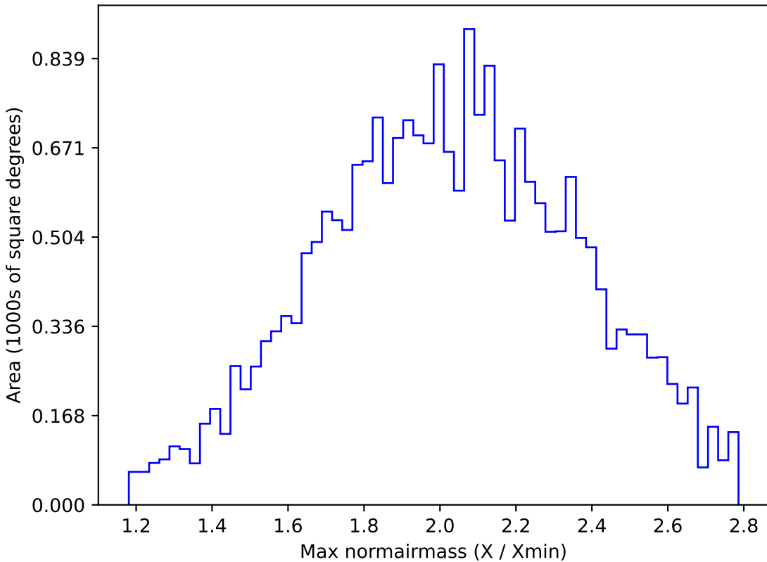
baseline_v3.2_10yrs All sky y band: Max normairmass
