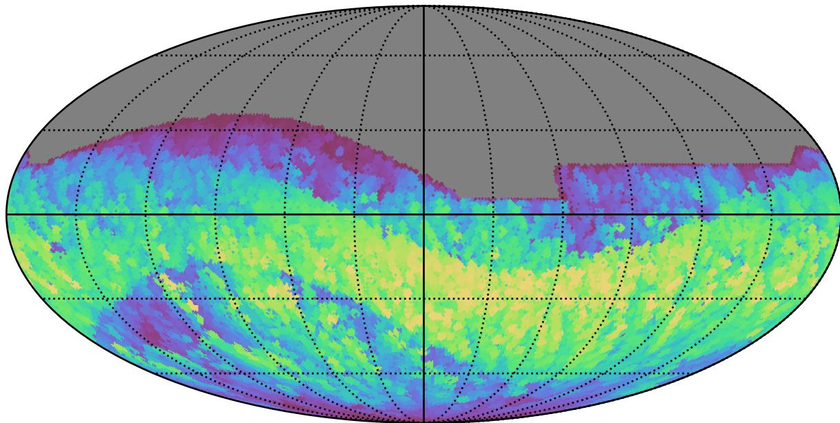
baseline_v3.2_10yrs All sky i band: Max normairmass
