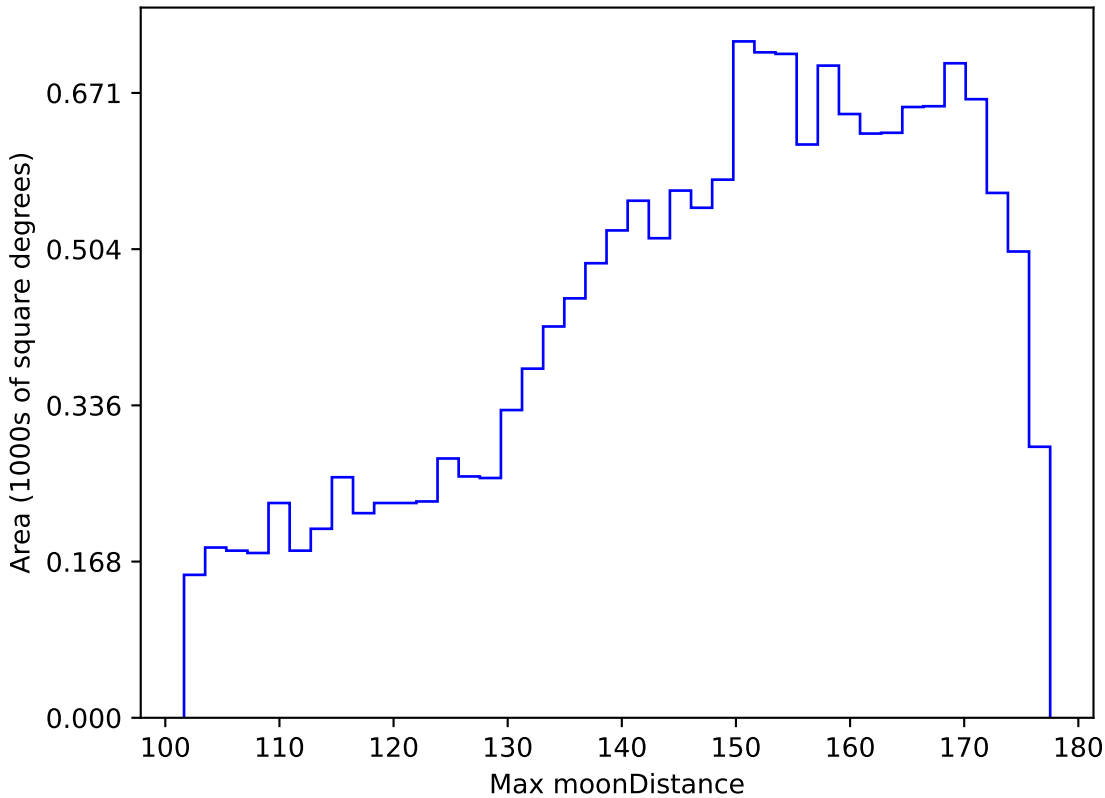
baseline_v3.2_10yrs WFD y band: Max moonDistance
