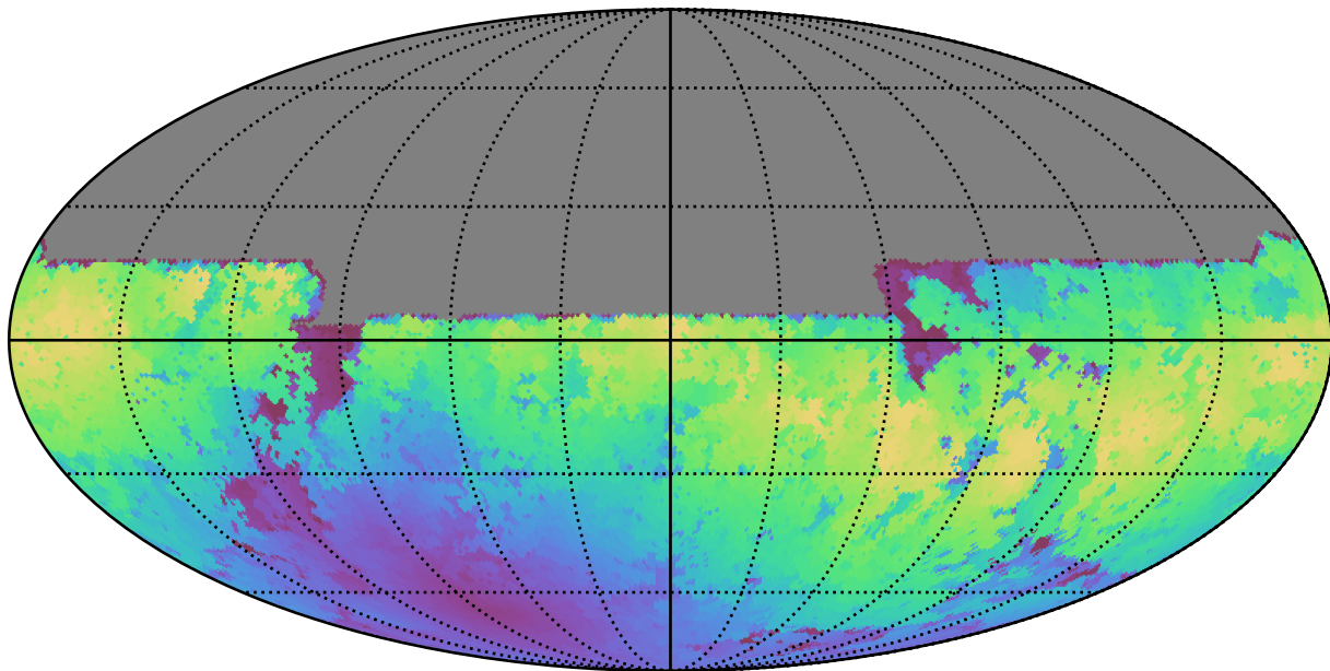
baseline_v3.2_10yrs All sky y band: Max moonDistance
