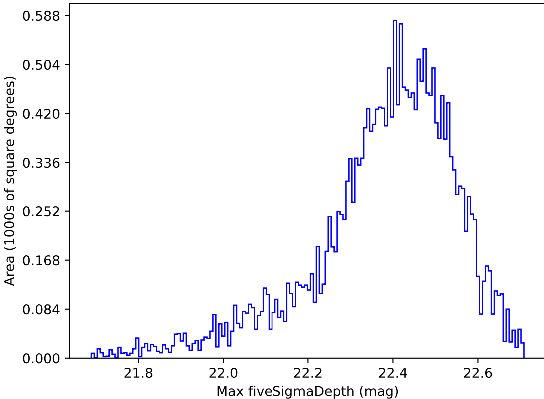
baseline_v3.2_10yrs Yr 1 y band: Max fiveSigmaDepth
