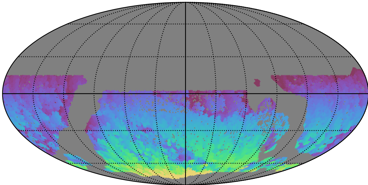
baseline_v3.2_10yrs WFD z band: Max HA
