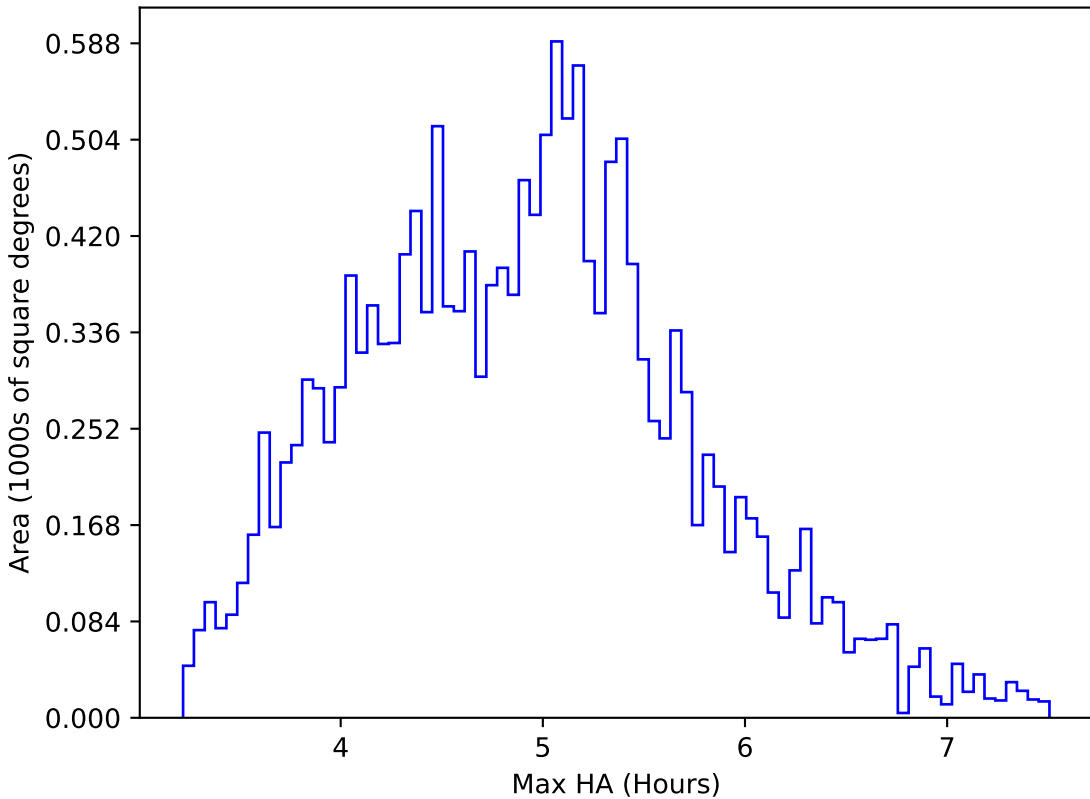
baseline_v3.2_10yrs WFD z band: Max HA
