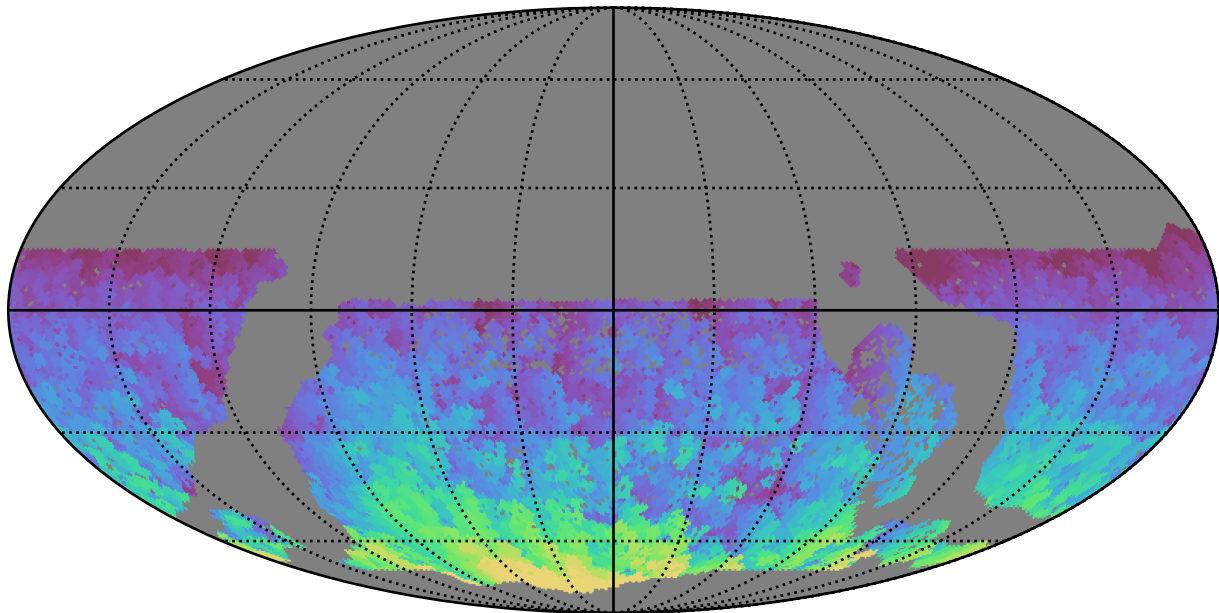
baseline_v3.2_10yrs WFD y band: Max HA
