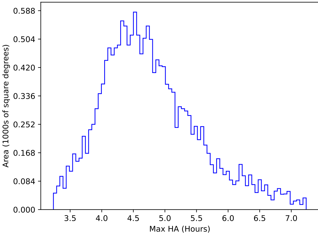
baseline_v3.2_10yrs WFD y band: Max HA
