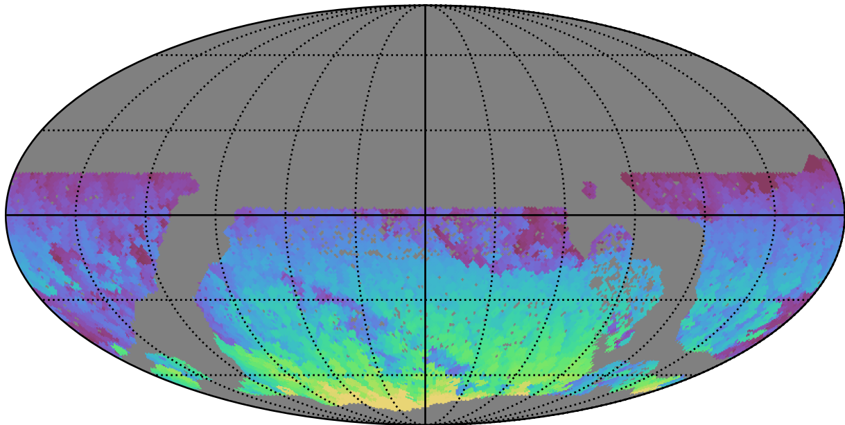
baseline_v3.2_10yrs WFD i band: Max HA
