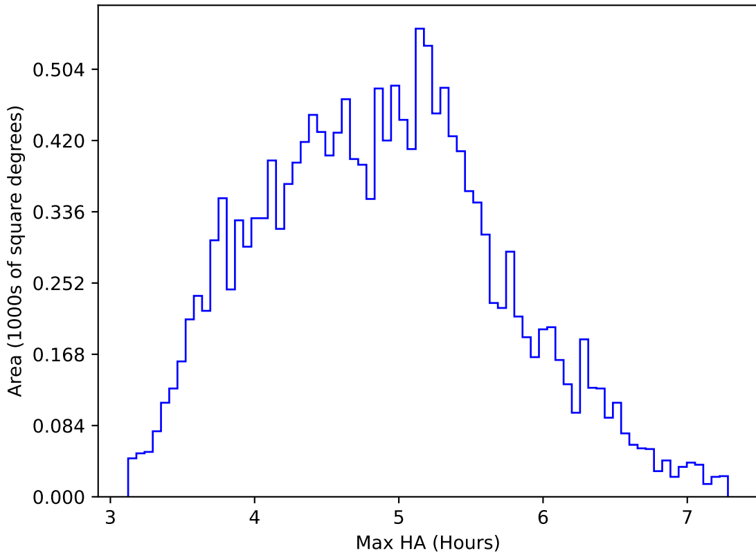
baseline_v3.2_10yrs WFD i band: Max HA
