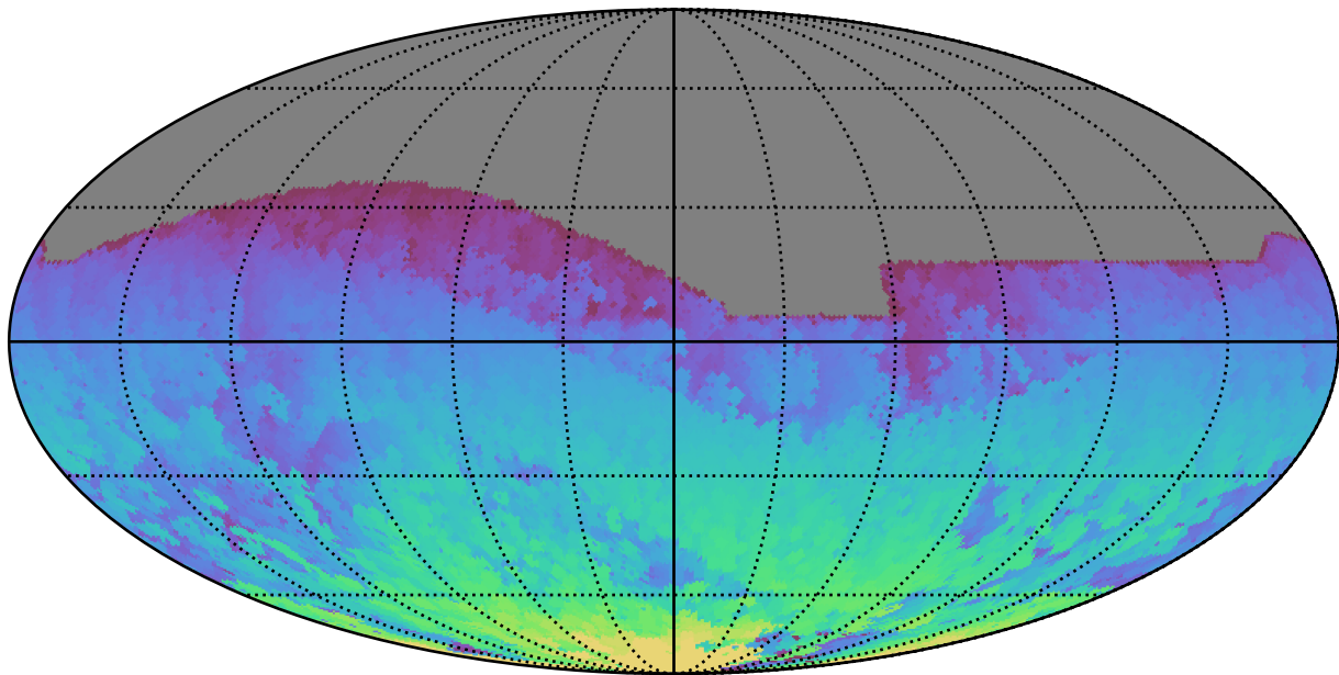
baseline_v3.2_10yrs All sky z band: Max HA
