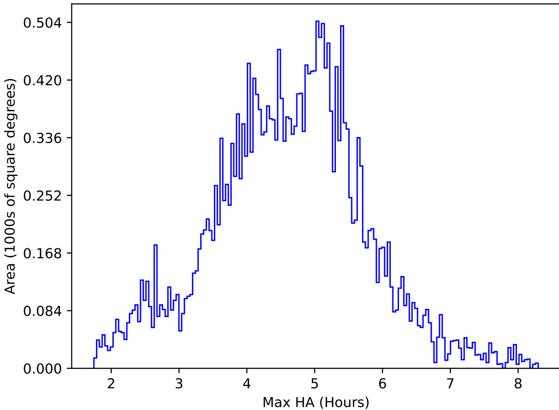
baseline_v3.2_10yrs All sky z band: Max HA
