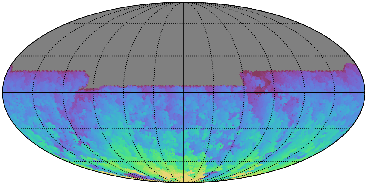
baseline_v3.2_10yrs All sky y band: Max HA
