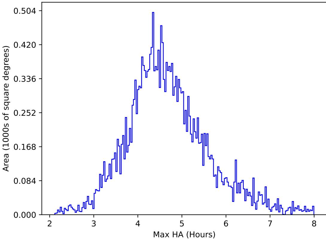
baseline_v3.2_10yrs All sky y band: Max HA
