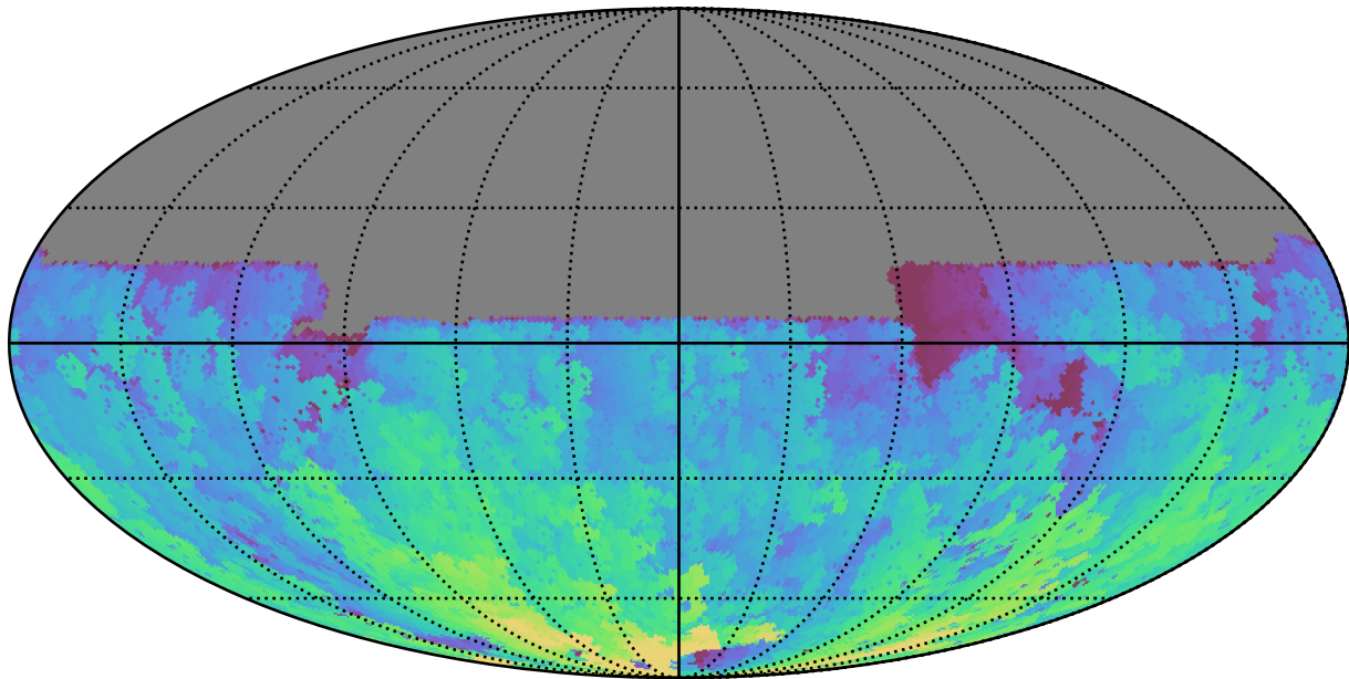
baseline_v3.2_10yrs All sky u band: Max HA
