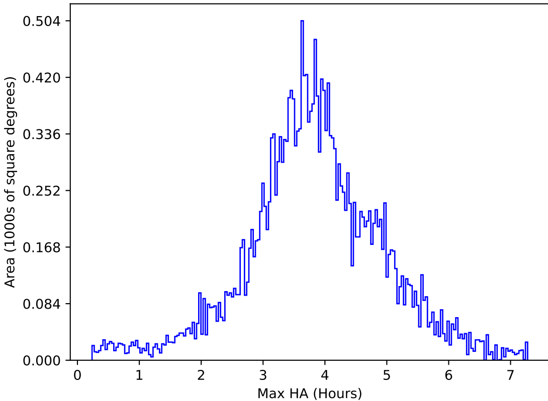
baseline_v3.2_10yrs All sky u band: Max HA
