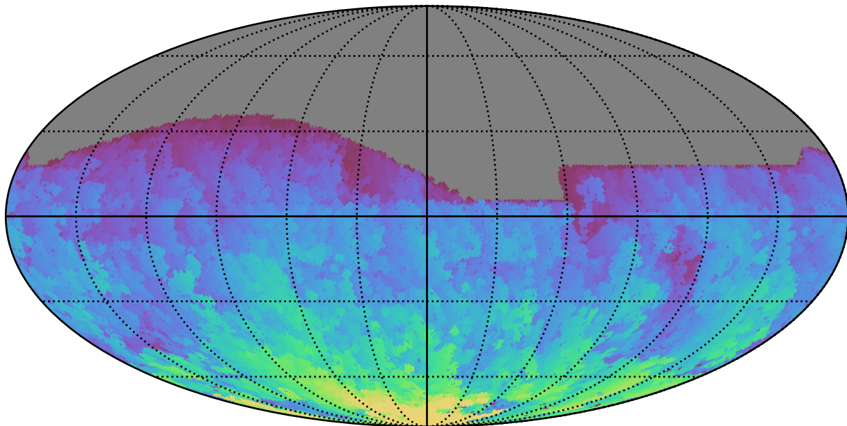
baseline_v3.2_10yrs All sky r band: Max HA
