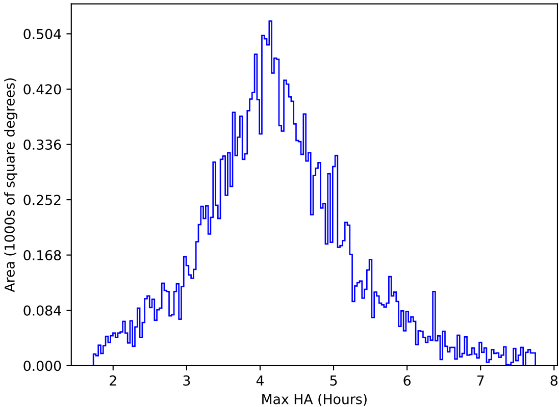
baseline_v3.2_10yrs All sky r band: Max HA
