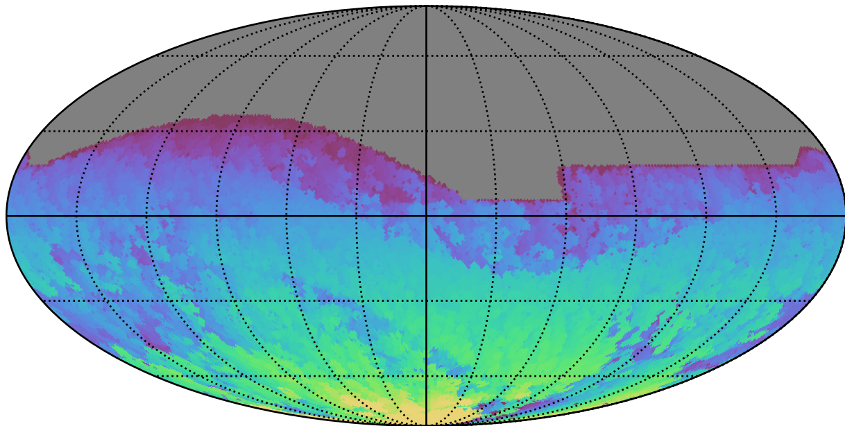
baseline_v3.2_10yrs All sky i band: Max HA
