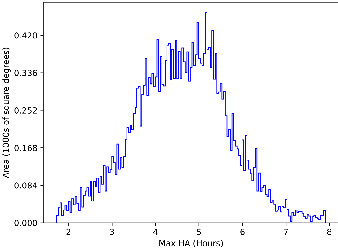
baseline_v3.2_10yrs All sky i band: Max HA
