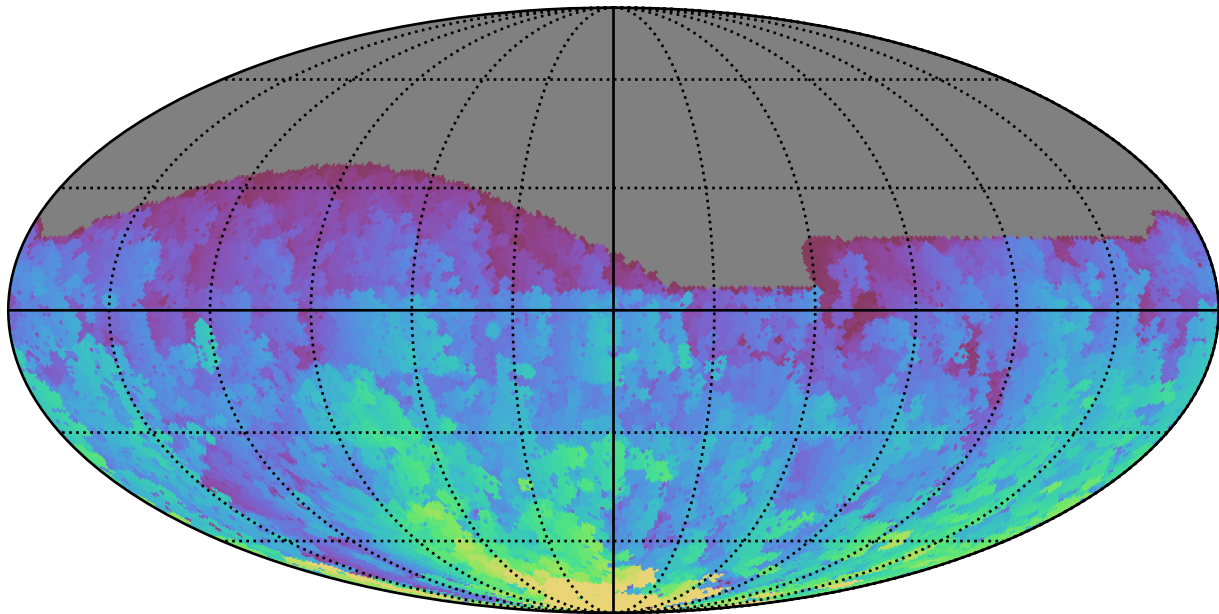
baseline_v3.2_10yrs All sky g band: Max HA
