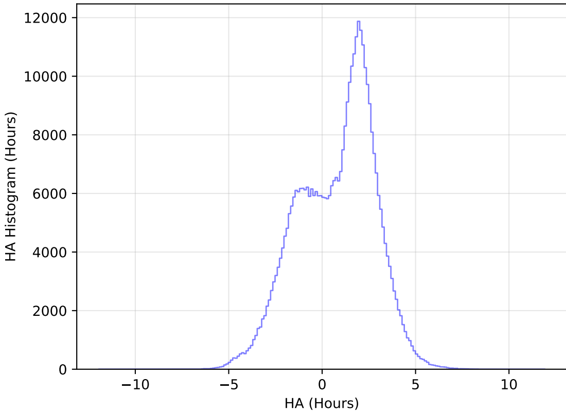
baseline_v3.2_10yrs All sky y band: HA Histogram
