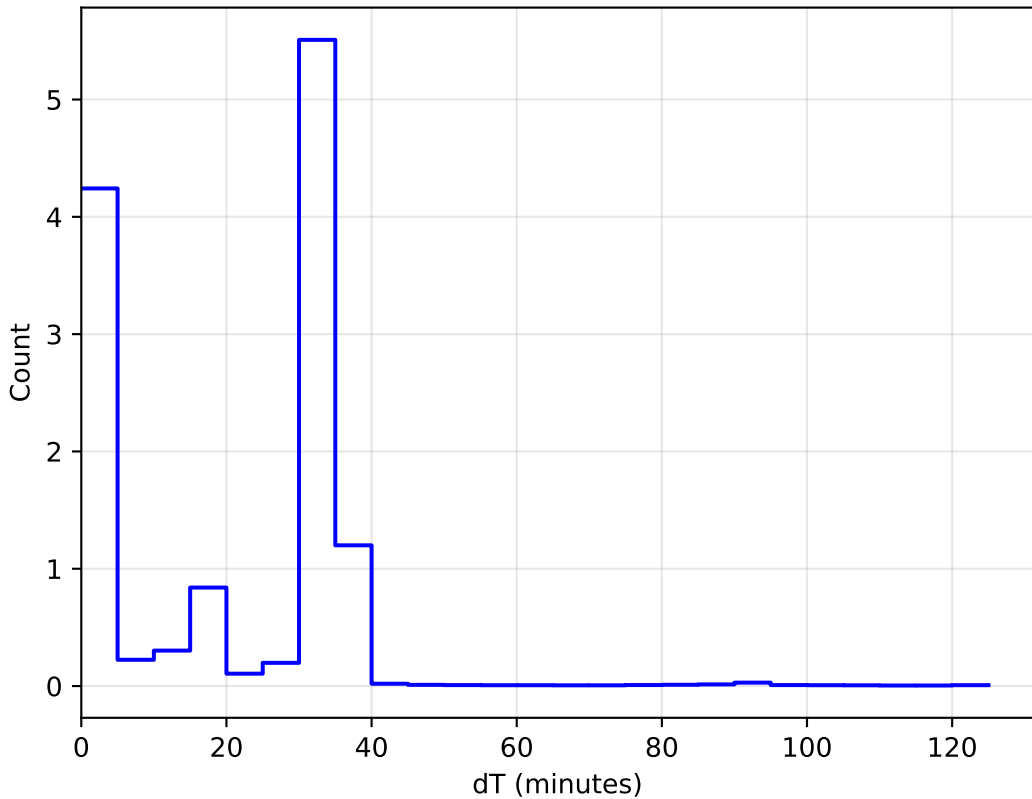
1e6 baseline_v3.2_10yrs All sky: DeltaT Histogram
