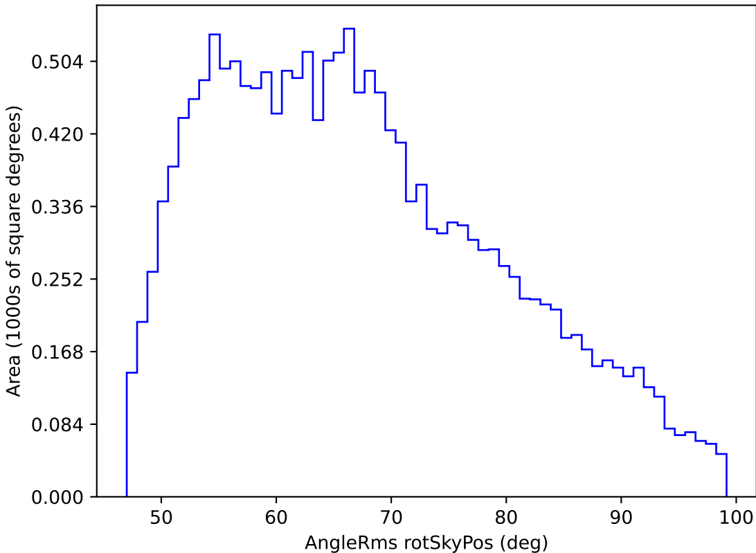
baseline_v3.2_10yrs WFD y band: AngleRms rotSkyPos
